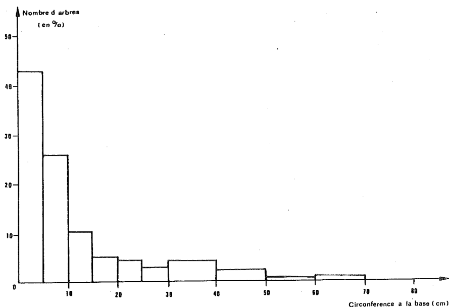
Figure 1 : Répartition d' Acacia senegal en fonction de la longueur de la circonférence.
