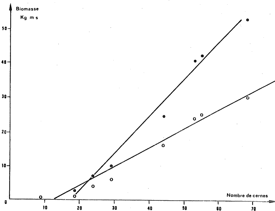
Figure 5 : Biomasse du tronc et des branches en fonction du nombre de cerne.
