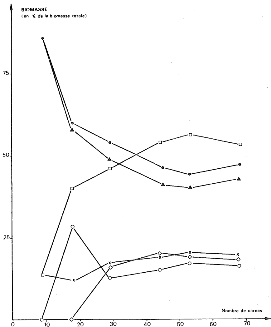
Figure 12 : Répartition de la biomasse ligneuse d' Acacia senegal en fonction du nombre de cerne.
