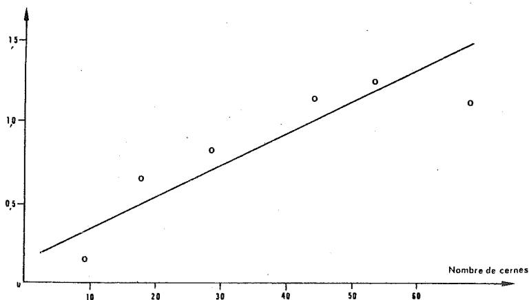
Figure 10 : Evolution de \lambda en fonction du nombre de cernes.
